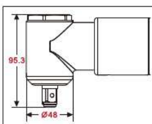
OP-100LH 1/2" Rear exhaust 後排氣
